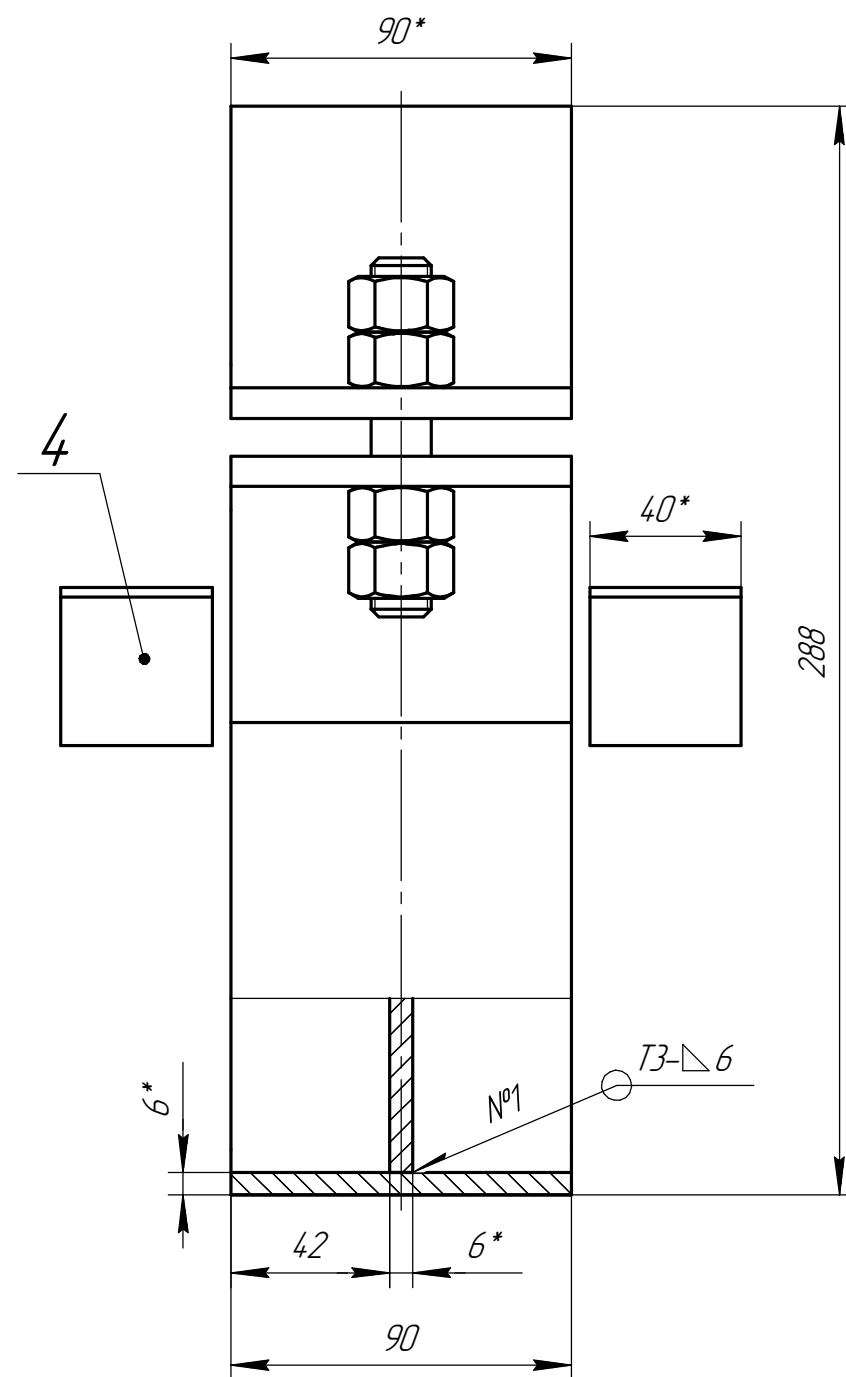
Det. poz. 1 (1:2)
