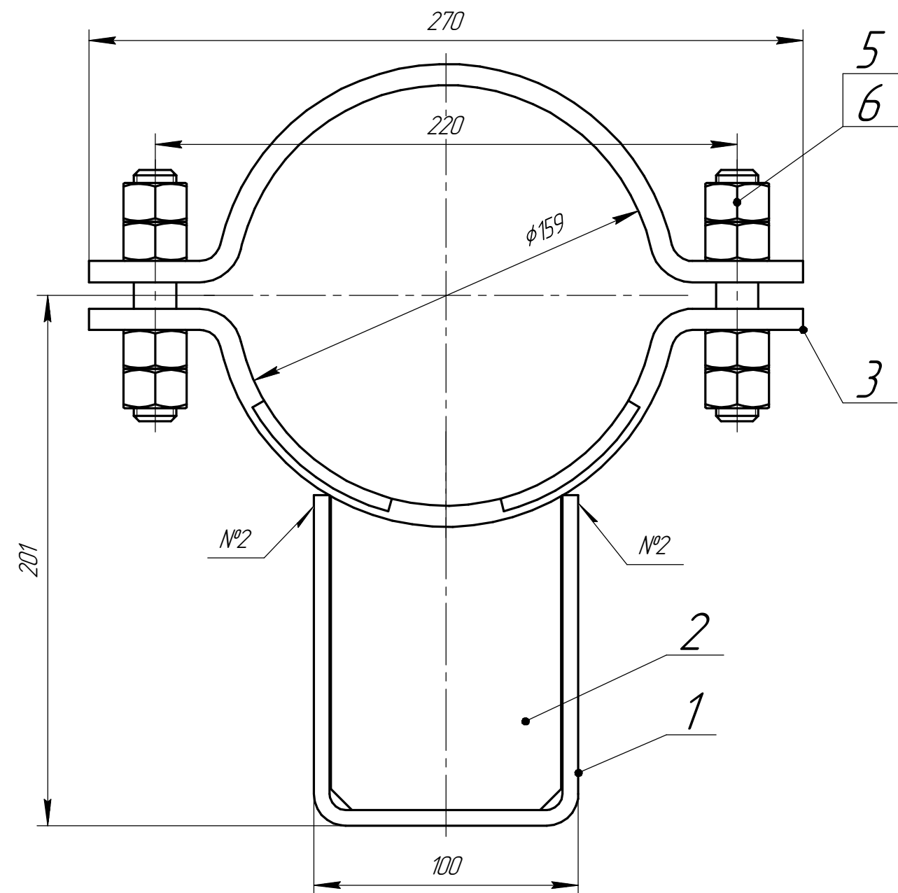
Det. poz. 3
