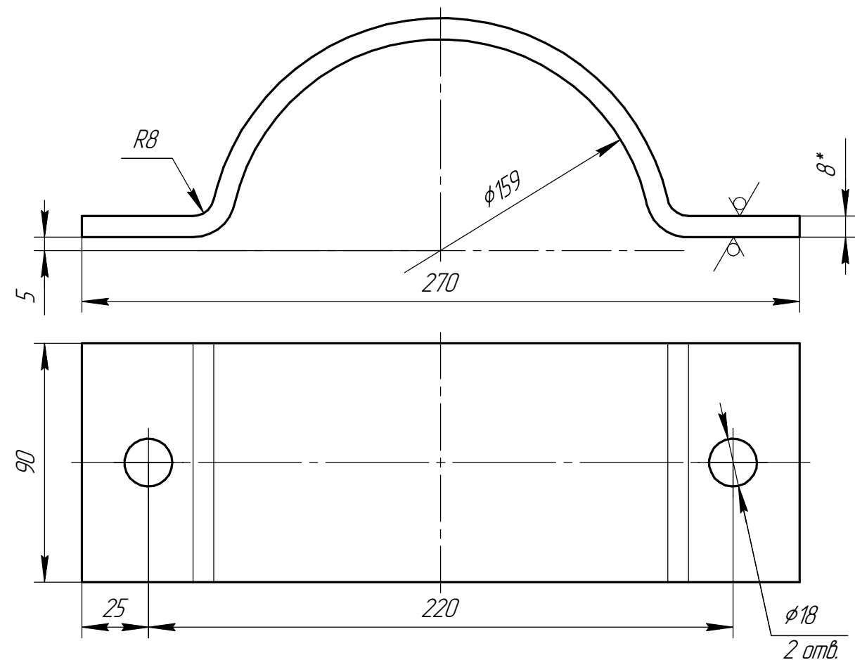
Det. poz. 3
