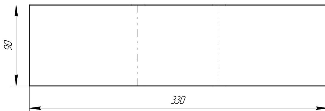
Q (1:2,5)
